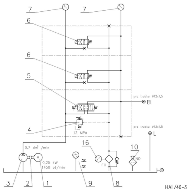
obrázek: Schéma elektro- hydraulického systému regulace Točivé redukce
